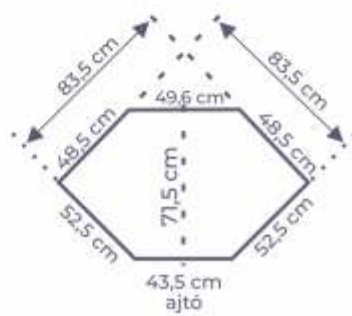
Bern sarokelem belső elrendezés
